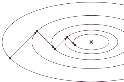
Рис. 1: Наискорейший спуск.
