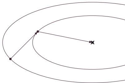
Рис. 2: Сопряжённые градиенты.
